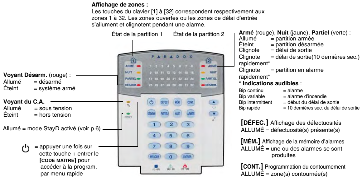
Figure 2 : MG32LED (clavier à DEL pour 32 zones)
