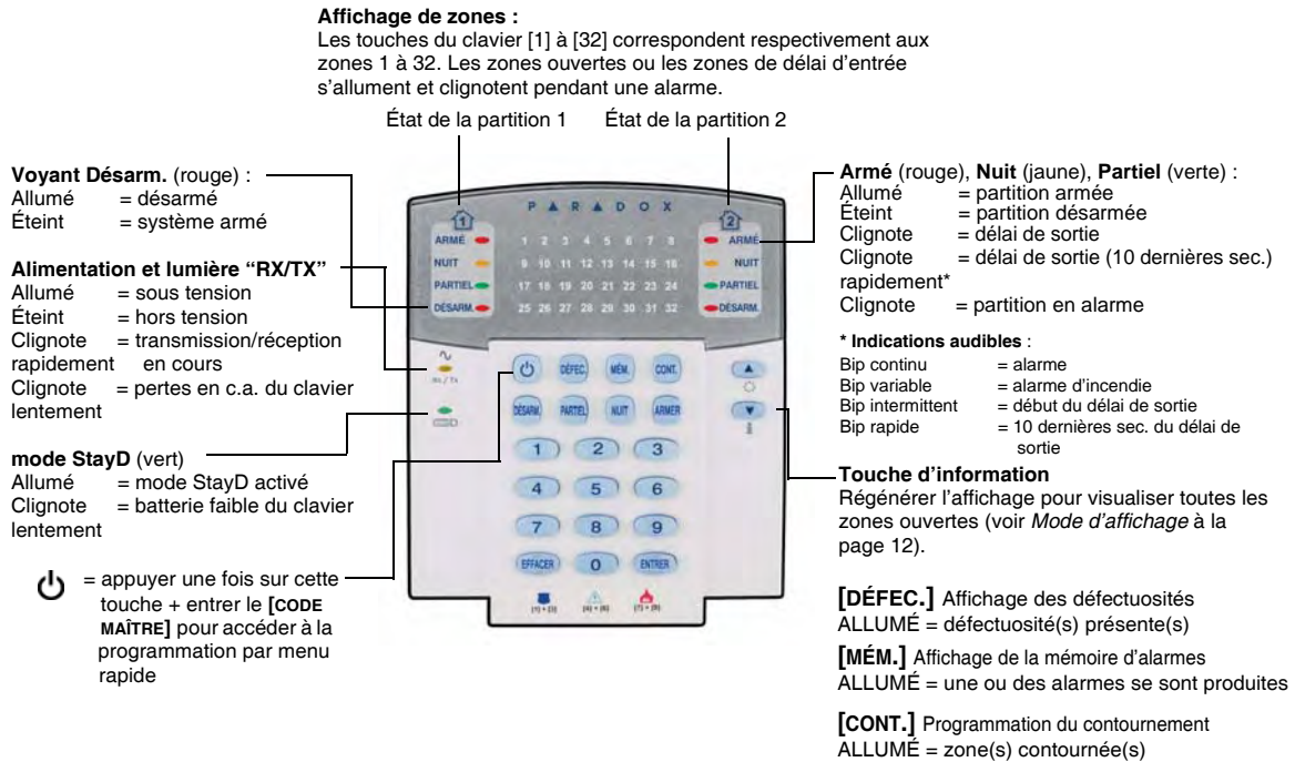
Figure 3 : MG32LRF (clavier à DEL pour 32 zones)
